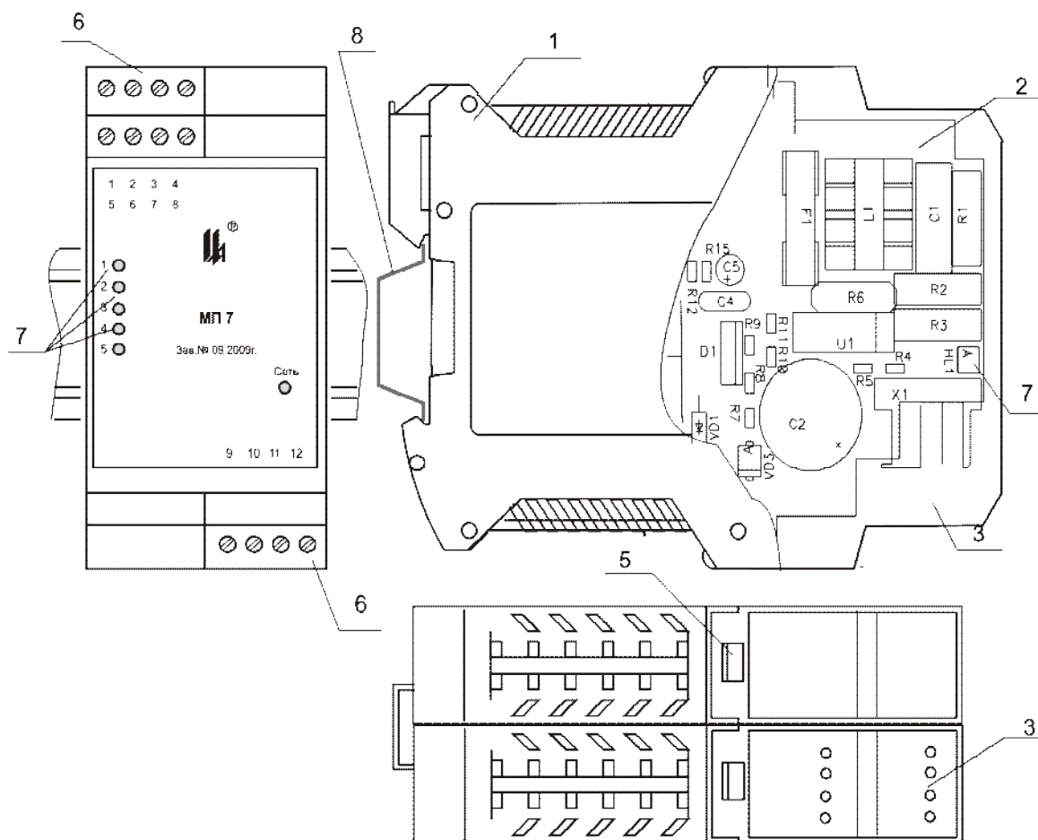
Рисунок 4.1 – Конструкция МП-7
