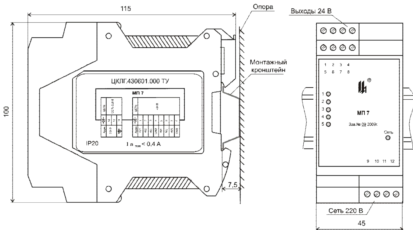
Рисунок 2.1 – Установочные размеры МП-7
